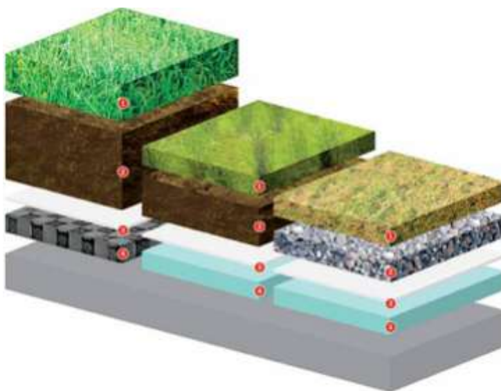
Στρωμάτωση εντατικού, ημιεντατικού και εκτακτικού τύπου φύτευσης πράσινης ταράτσας
