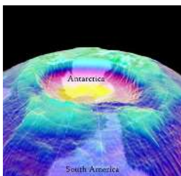
Η τρύπα του Όζοντος στην Ανταρκτική
