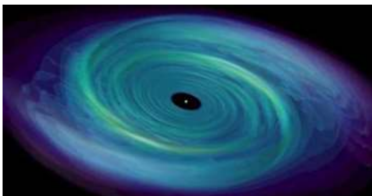
Μαύρη τρύπα στο κέντρο του γαλαξία M87
